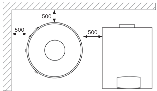
Abb. 1 Speicheraufstellung im Installationsraum
