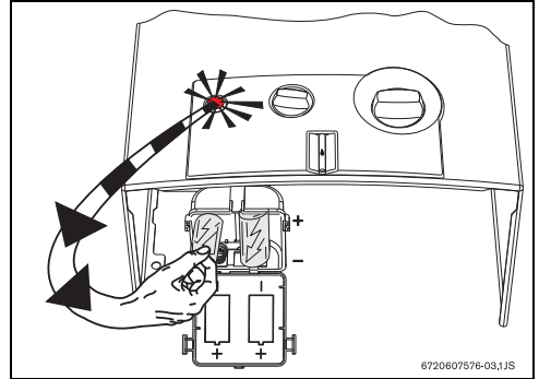
Bild 5 Ersetzen der Batterien
