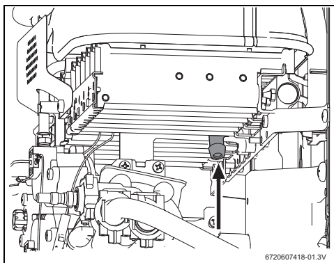
Bild 13 Messpunkt für den Druck
