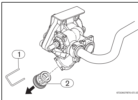
Bild 15 Entlüften
