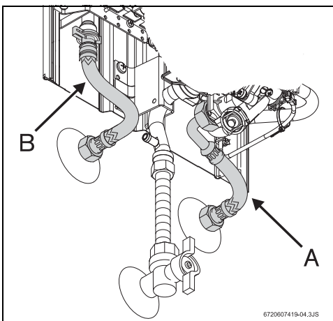
Bild 12 Wasseranschluss
