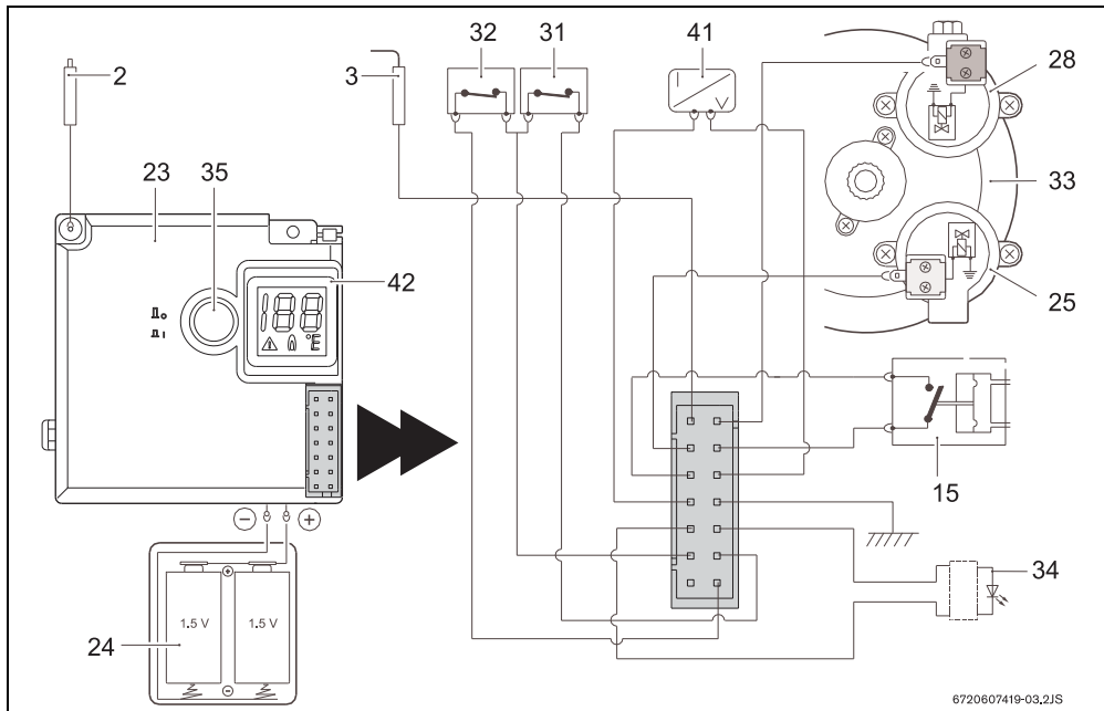
Bild 2 Schaltplan
