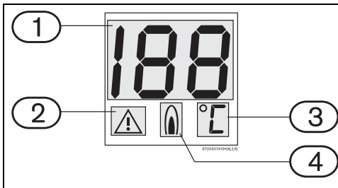
Bild 3 Digitalanzeige
