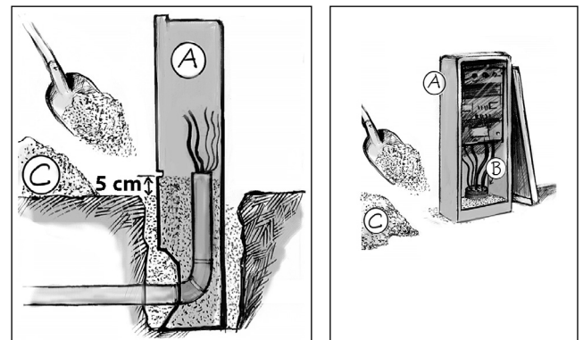
A=Apparatskåp, B=Avtätning, C=Torr vit sand.
