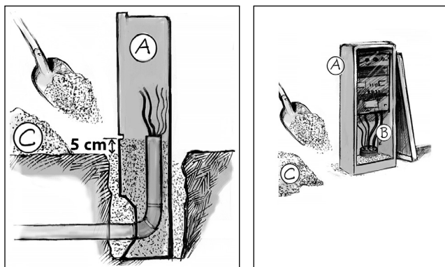
A-prázdnne teleso B-tesniaca zátka C-suchý biely piesok
