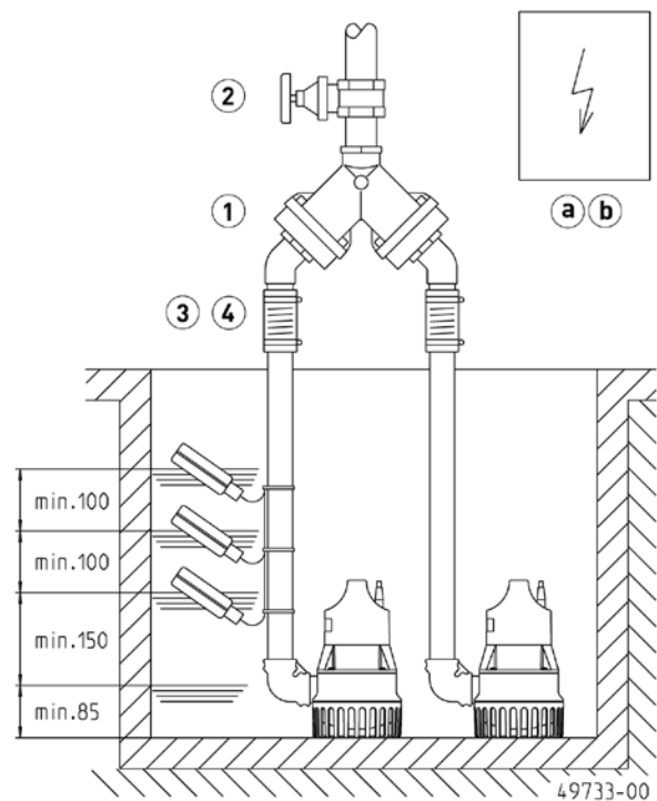
Einbaubeispiel Doppelanlage
