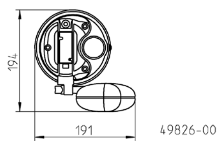
Einbaubeispiel Doppelanlage
