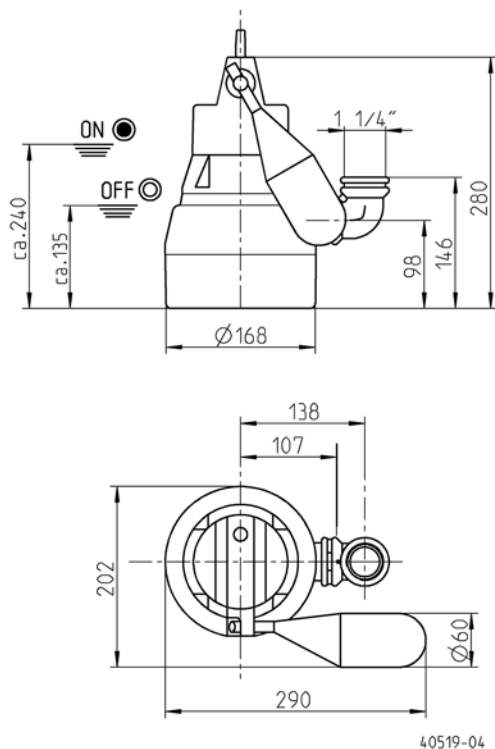
Hauptmaße und Schalthöhen U5KS (mm)
