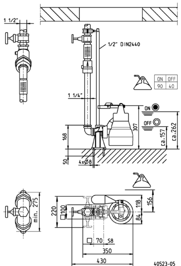
Hauptmaße und Schalthöhen GR 32 (mm)
