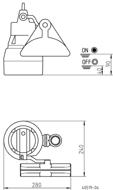
Hauptmaße und Schalthöhen Sonderschwimmer (mm)
