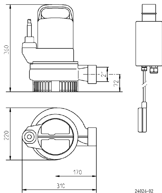
Hauptmaße US 151 und US 251 (mm)
