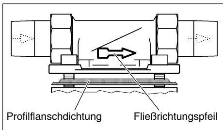
Abb. 2: Einbaudrehflansch
