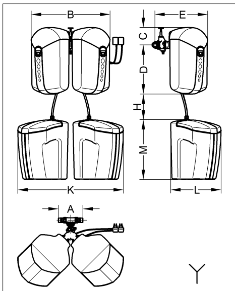
Abb. 16: Einbaumaße
