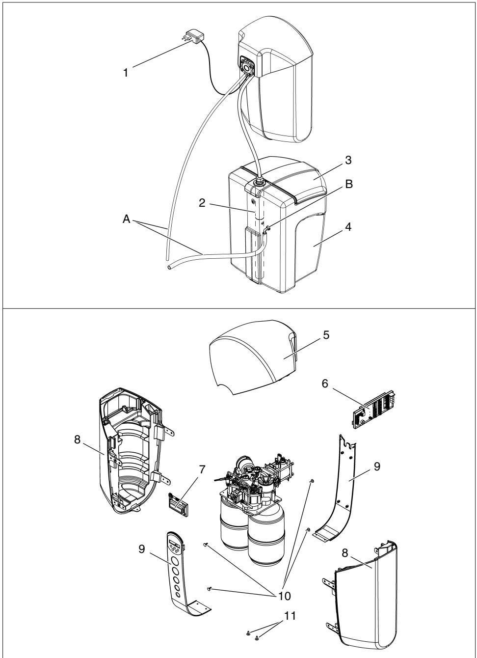
Abb. 18: Ersatzteile JUDO SOFTwell MEGA 4
