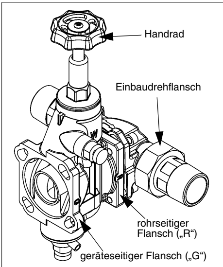
Abb. 3: Umgehungsventil (JQX)
