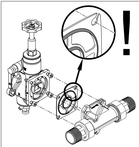
Abb. 4: Profilflanschdichtung
