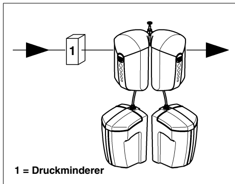
Abb. 1: Druckminderer vor der Anlage
