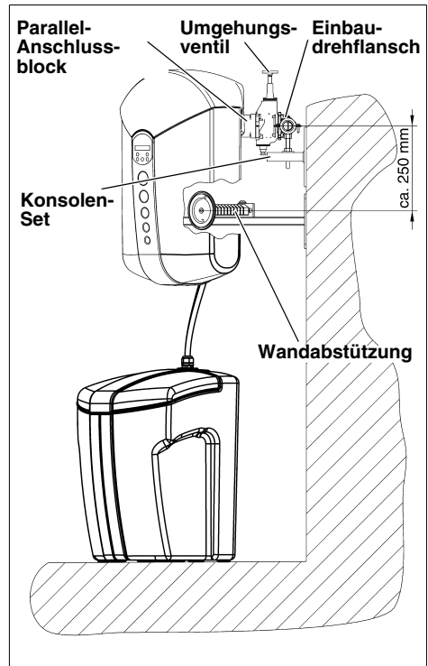
Abb. 5: Abstützungselemente
