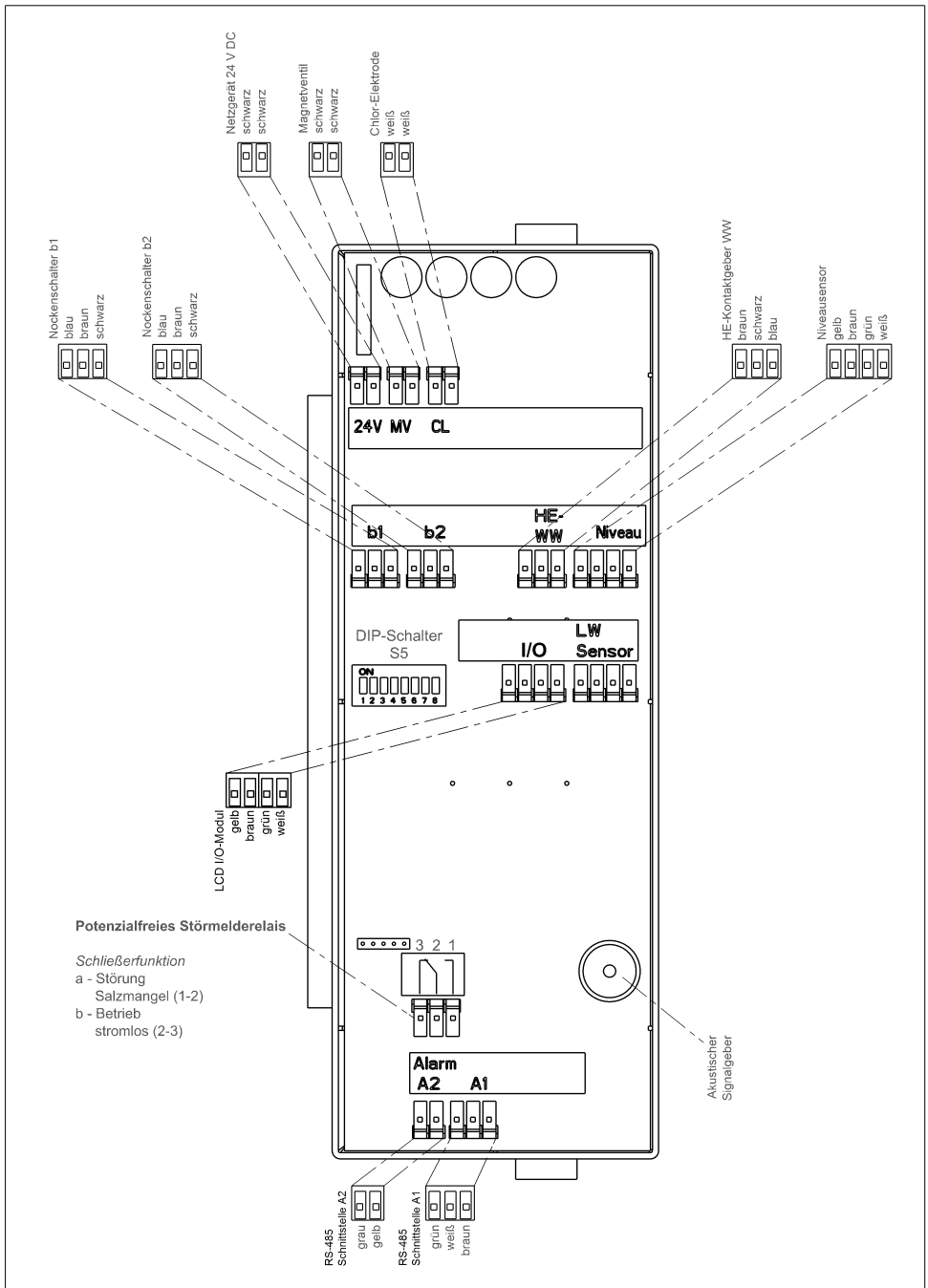
Abb. 17: Elektronische Steuerung mit Störmelderelais
