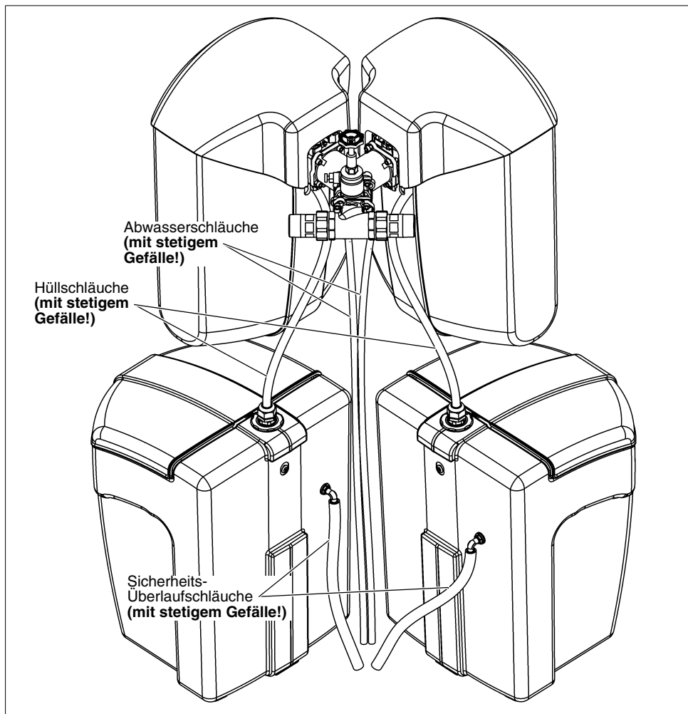
Abb. 10: Anschluss an Siphon
