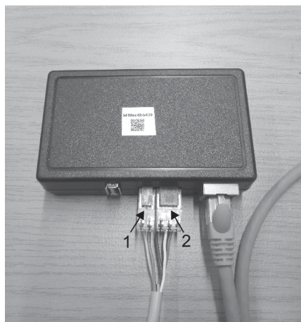
Afb. 4: Kabel aansluiting aan connectivity-module
