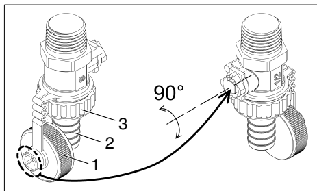
Abb. 8: Sicherheits-Kugelhahn
