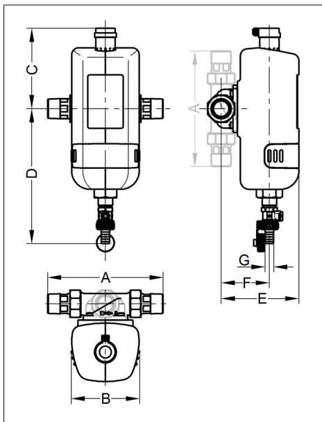
Abb. 10: Einbaumaße JMFI 3/4" - 1 1/4"
