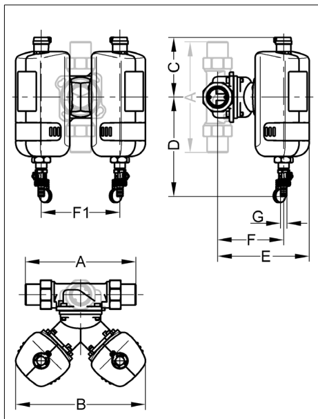
Abb. 11: Einbaumaße JMFI 1 1/2"
