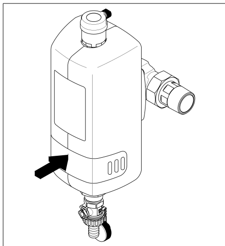
Abb. 9: Magnethalter einschieben
