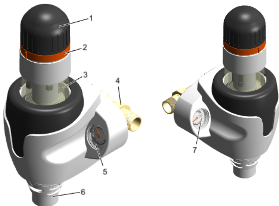
Abb. 1: Funktionsbeschreibung
