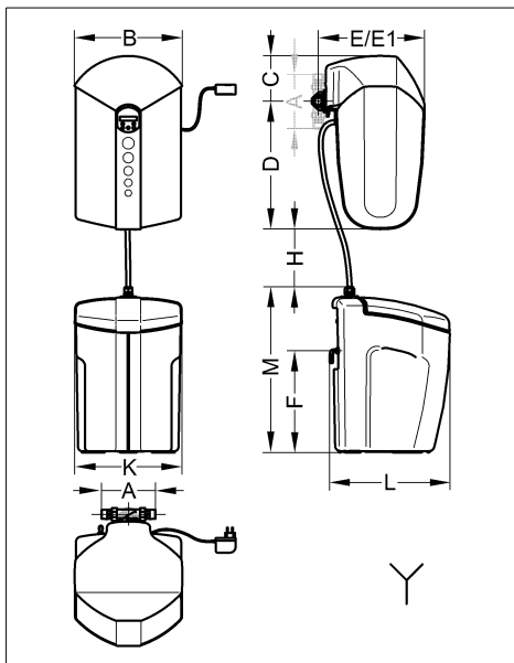
Abb. 19: Einbaumaße
