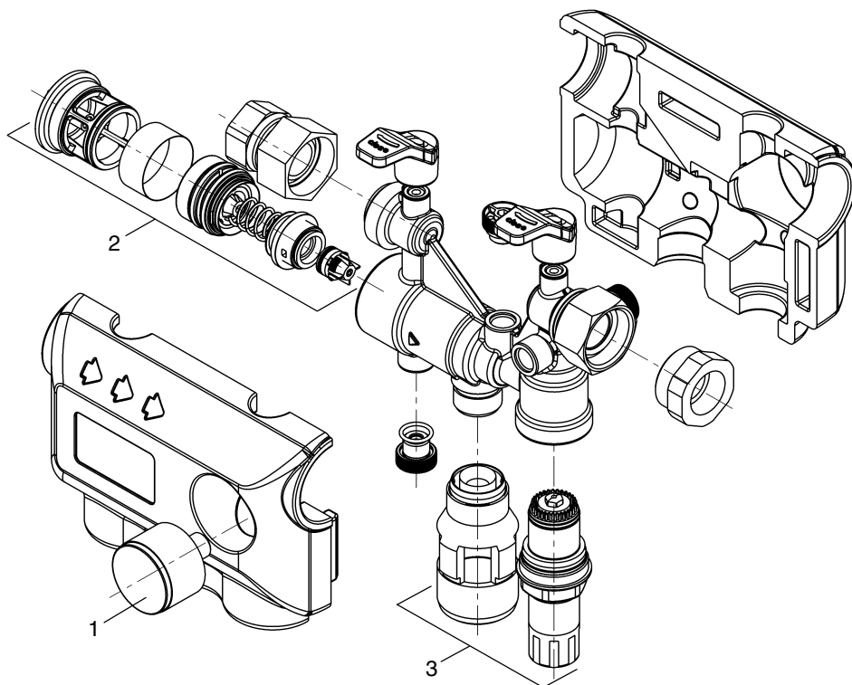
Ersatzteilliste JHF-F PLUS ¾"
