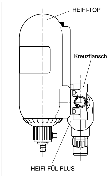
Abb. 1: JHF-K PLUS Seitenansicht
