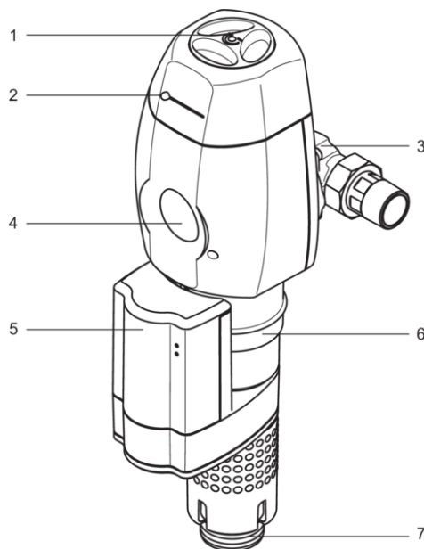
Abb. 1: Funktionsbeschreibung
