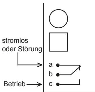
Abb. 10: Belegung Relaiskontakte
