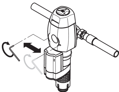
Abb. 6: Festschrauben JUKOMAT-EC-AT
