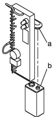
Abb. 9: Batteriewechsel
