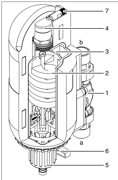
Fig. 10: Description fonctionnelle
