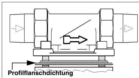
Abb. 5: Einbaudrehflansch
