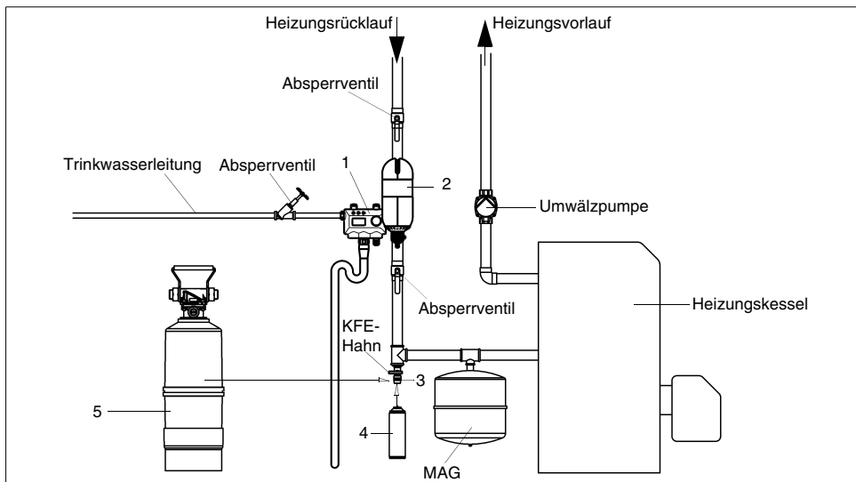
Abb. 2: Schema JUDO HEIFI-TOP mit mobiler Heizungswasseraufbereitung nach VDI 2035
