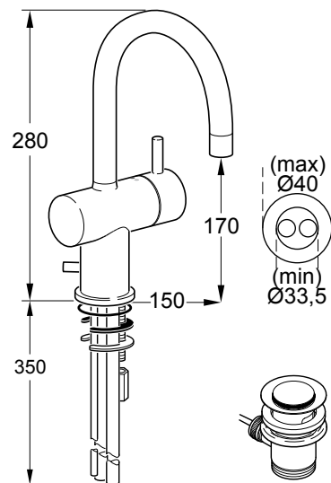
Einhebel-Waschtisch-Batterie, mit Ab- und Überlauf verchromt F1276AA
