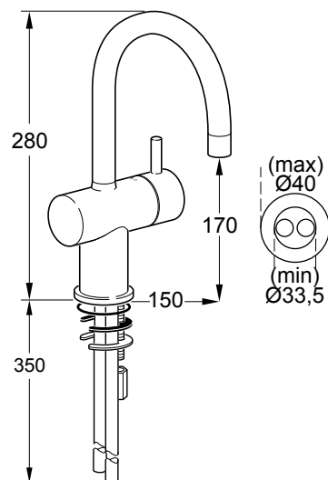
Einhebel-Waschtisch-Batterie, ohne Ab- und Überlauf verchromt F1277AA
