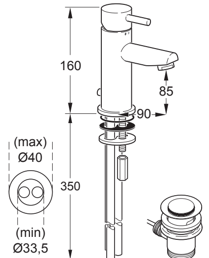
Waschtiszbatterie mit Ab- und Überlauf verchromt F1269AA Waschtiszbatterie ohne Ab- und Überlauf verchromt F1271AA
