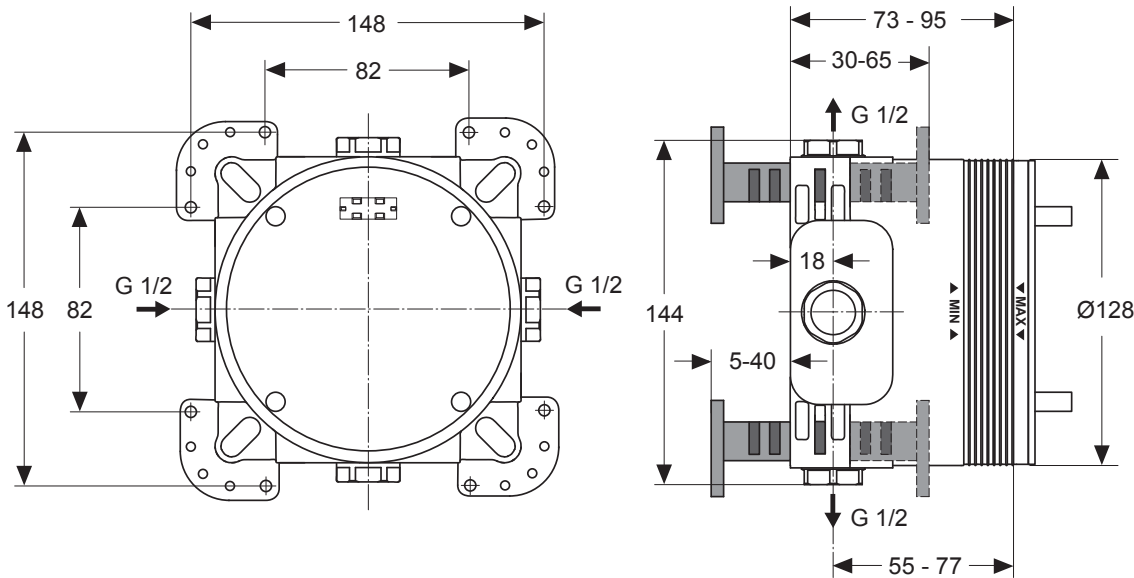
Unterputz-Bausatz 1 A1000NU
