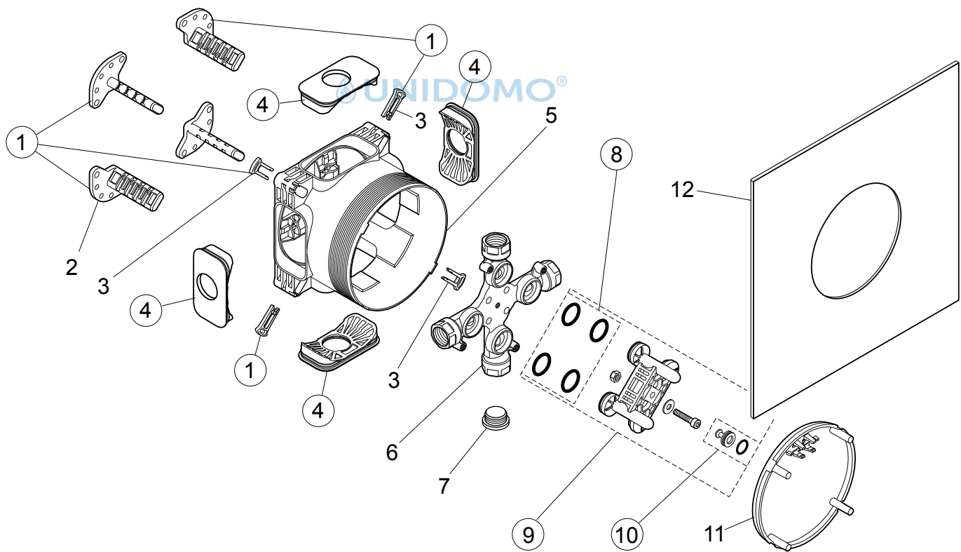
Unterputz-Bausatz 1 A1000NU
