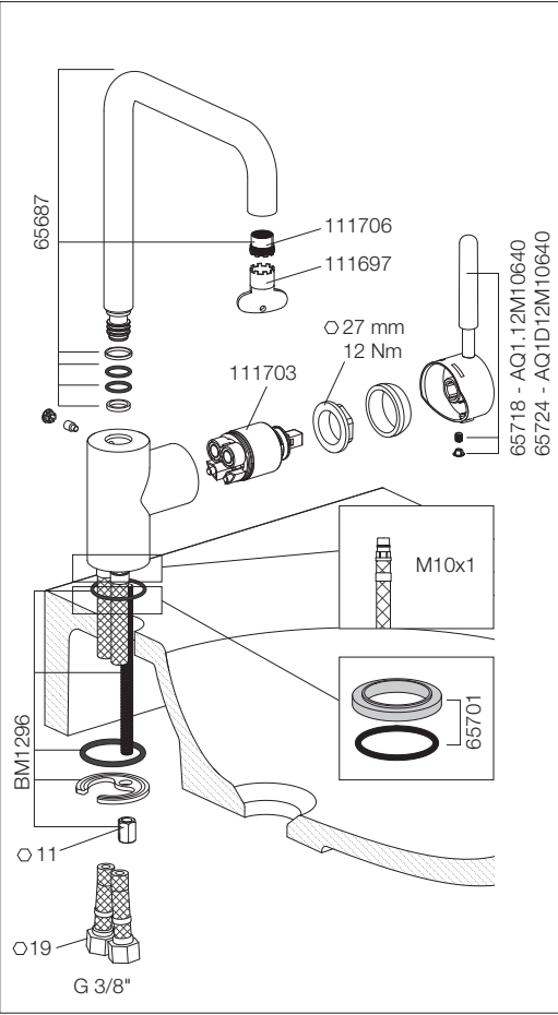
AQ1.12M10640 AQ1D12M10640
