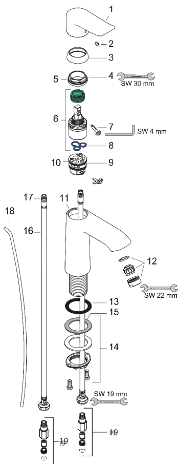
製品分解図
