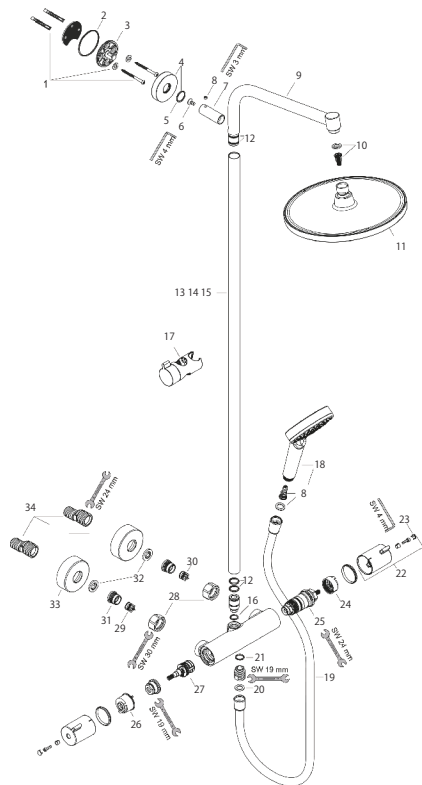
製品分解図
