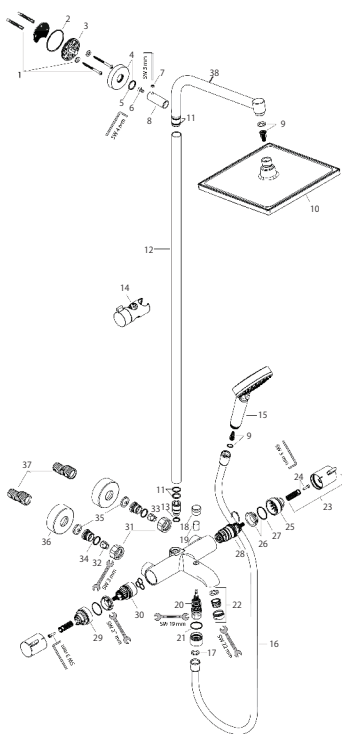
製品分解図
