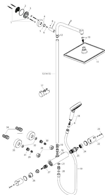
製品分解図
