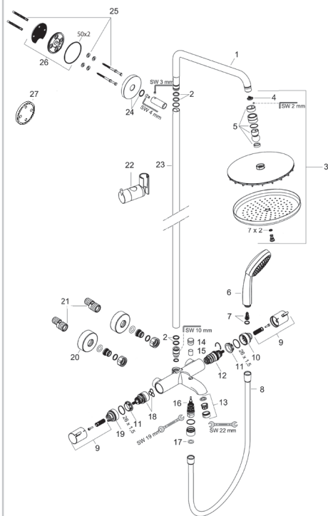
製品分解図
