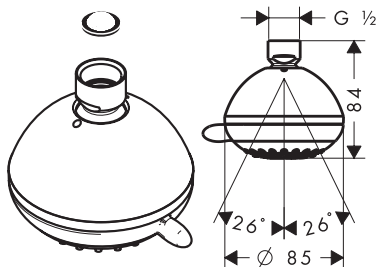
Crometta 85 Vario 28424000
