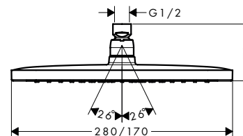
Croma E 280 1jet 26257000
