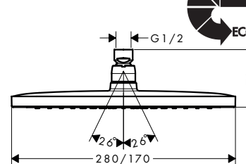
Croma E 280 1jet EcoSmart 26258000 / 26258007
