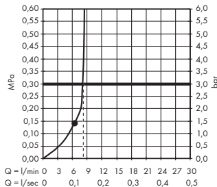
Croma E 280 1jet EcoSmart 26258000 / 26258007
