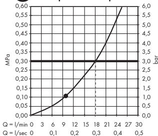
Croma E 280 1jet 26257000
