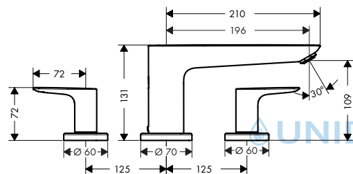
Talis E 71747000
