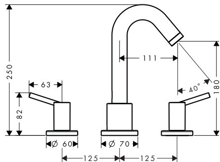
Talis S 32313000
