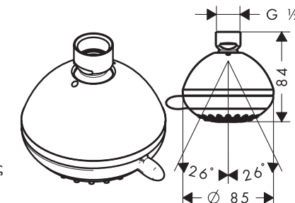
Crometta 85 Vario 28424000
