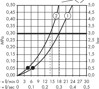
Crometta 85 Vario 28424000
