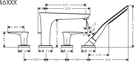
Metris S 31446000
