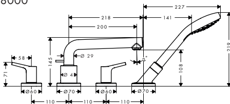
Talis S 72418000
