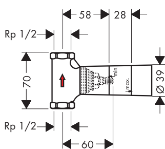
DN15 (1/2") 15973180
