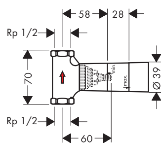
DN15 (1/2") 15974180
