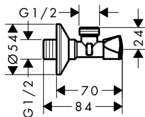
AXOR 51309000
