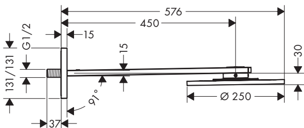
AXOR 250 1jet 35284XXX
