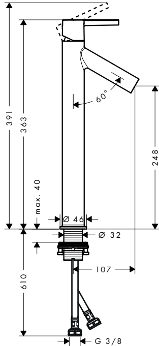
AXOR Starck 250 10103XXX
