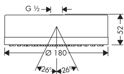
AXOR Citterio 28489000
