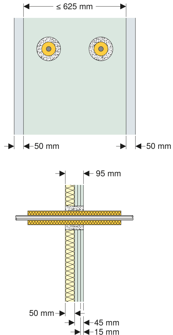
Abbildung 2: Dimensionierung Schachtwände
