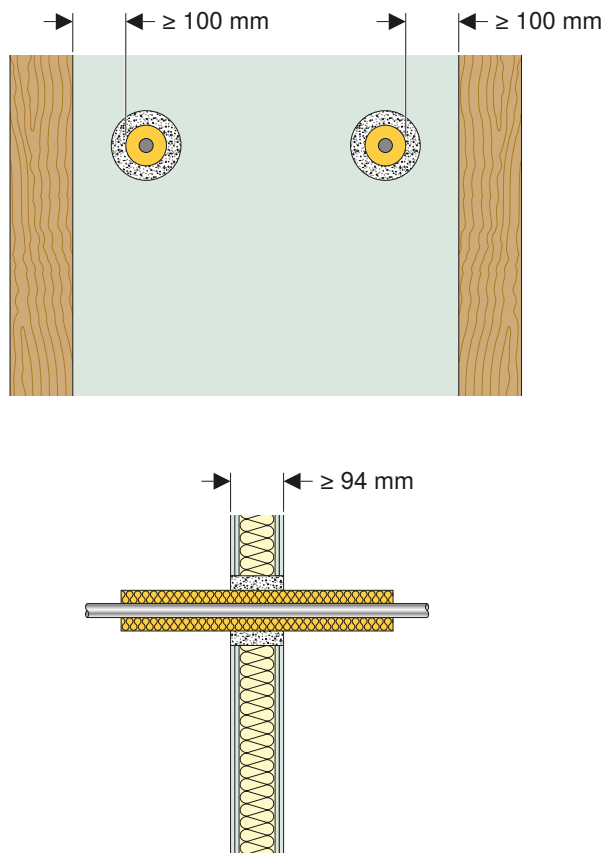
Abbildung 1: Dimensionierung Leichtbauwände
