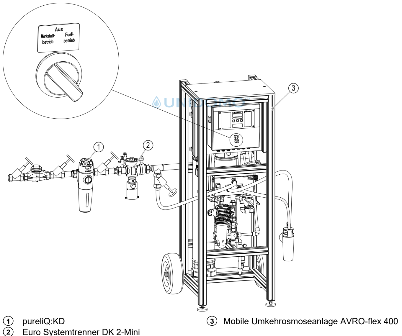
Abb. E-3: Installationszeichnung Mobile Umkehrosmoseanlage AVRO-flex 400 – Werkstattbetrieb
