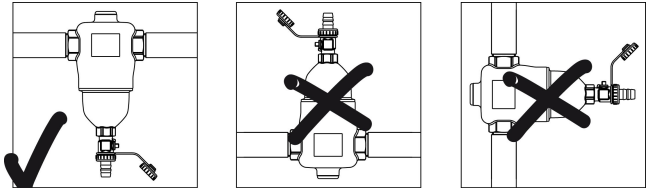
Abb. 3: Einbau Schlammabscheider
