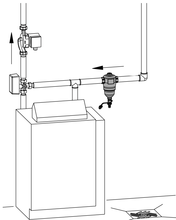
Abb. 4: Installationszeichnung Schlammabscheider
