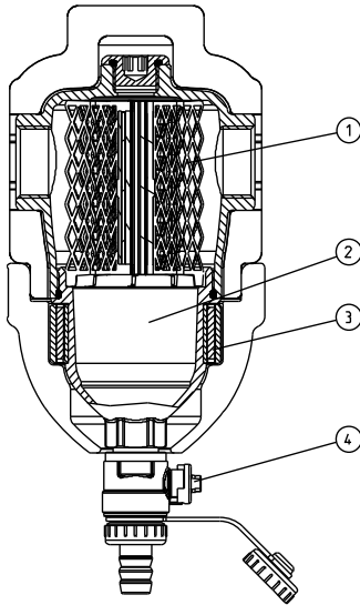
Abb. 2: Positionszeichnung
