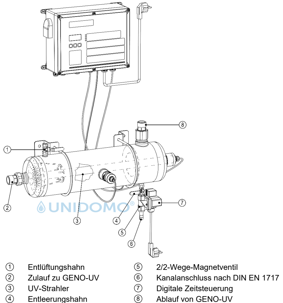
Abb. 1: Anlagenaufbau
