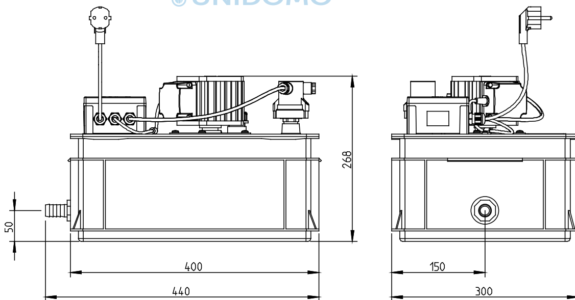
Abb.C-2: Maßzeichnung Abwasserhebeanlage AH-300
