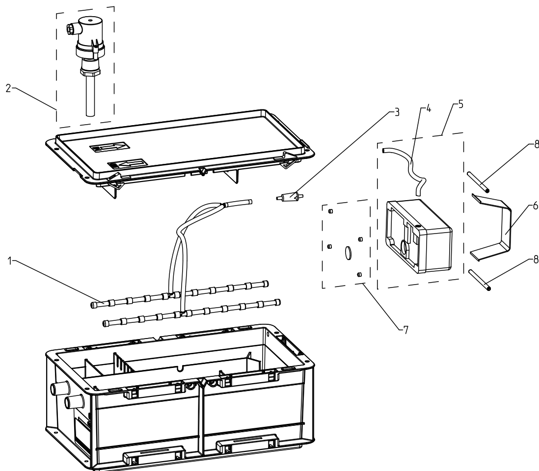
Abb. F-2: Verschleißteile GENO-Neutra NO-12
