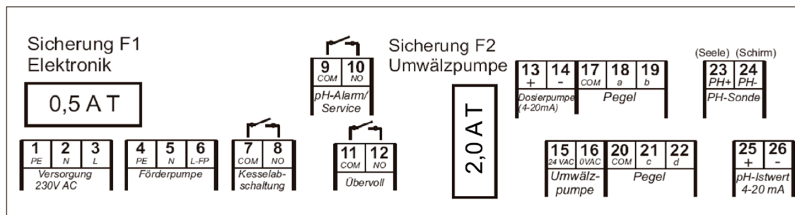
Abb. D-3: Klemmenbelegung der GENO-Neutra-matic 2
