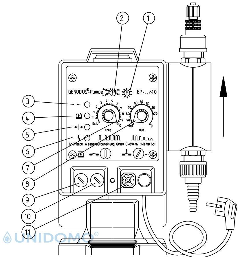
Abb. F-2: Betriebsarten GENODOS-Pumpe GP-.../40
