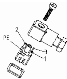
Abb. D-5: Anschluss-/Klemmenplan potentialfreie Sammelstörmeldung
