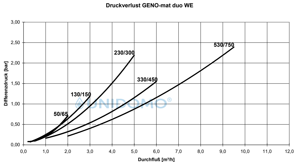
Abb. D-2: Druckverlustkurve GENO-mat duo WE
