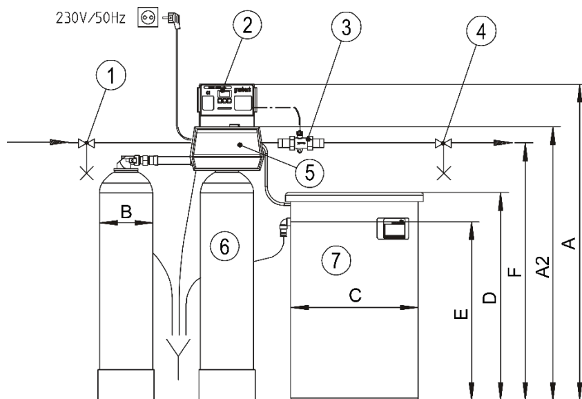
Abb. D-1 (a): Aufstellungszeichnung für Enthärtungsanlagen GENO-mat-duo WE
