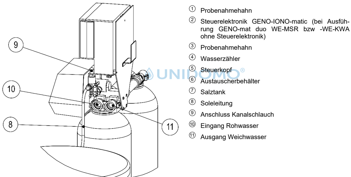
Abb. D-1 (b): Enthärtungsanlage GENO-mat-duo WE; Seitenansicht rechts/hinten
