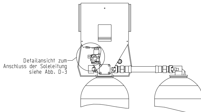
Abb. D-1 (b): Enthärtungsanlage GENO-mat-duo WE; Seitenansicht rechts/hinten
