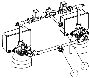
Abb. C-3 Verrohrung mit Magnetventilen
