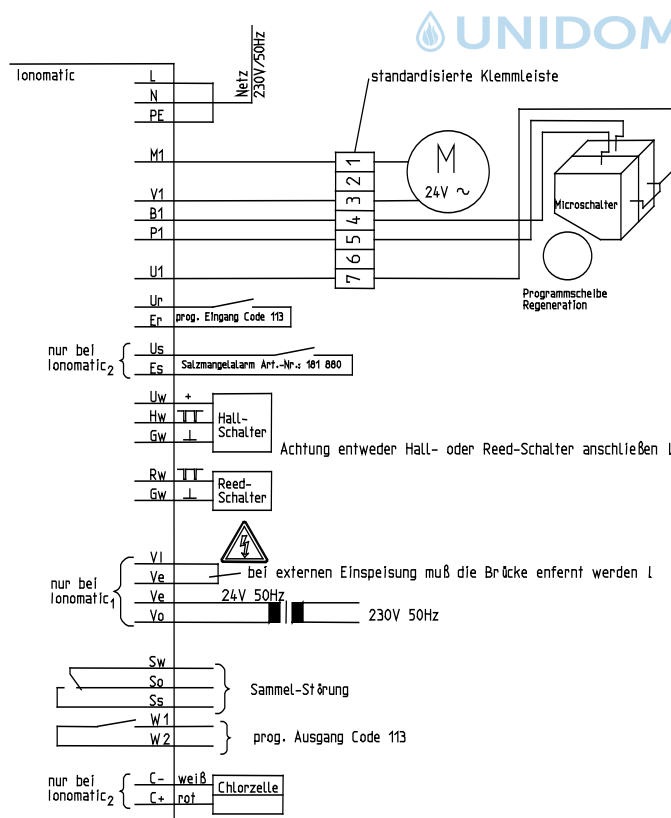
Abb. D-2: Klemmenanschlussplan GENO-mat-WF
