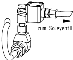
Desinfektionseinrichtung (vormontiert)
