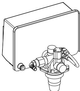
Abb. C-1: Steuerkopf Anschlussnennweite DN 25
