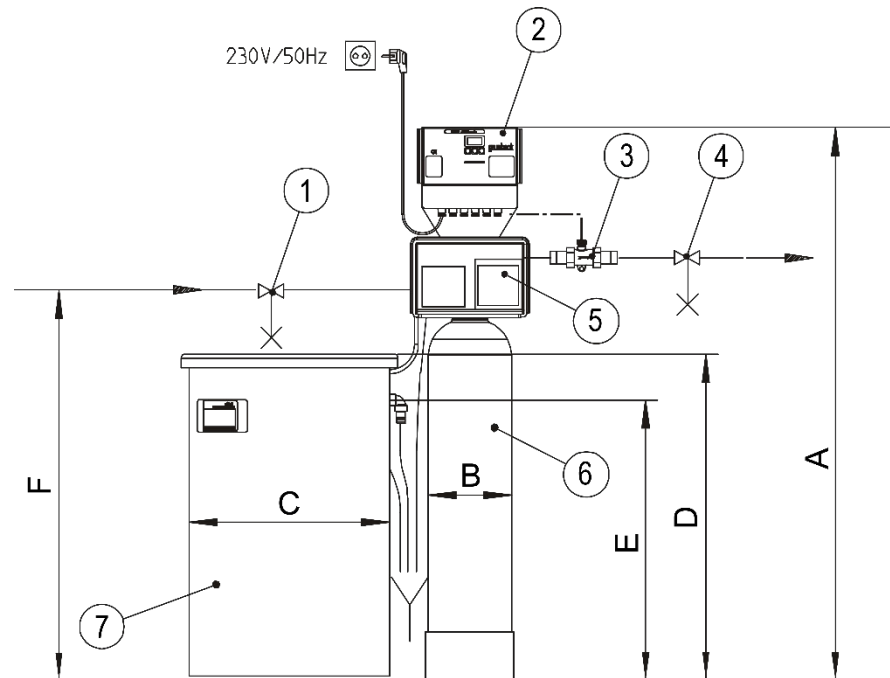
Abb. D-1: (a) Aufstellungszeichnung Enthärtungsanlage GENO-mat-WF
