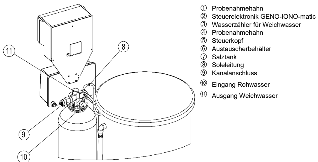
Abb. D-1: (b) Enthärtungsanlage GENO-mat-WF; Hinteransicht
