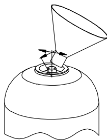
Steigrohr zentrieren, Harz einfüllen
