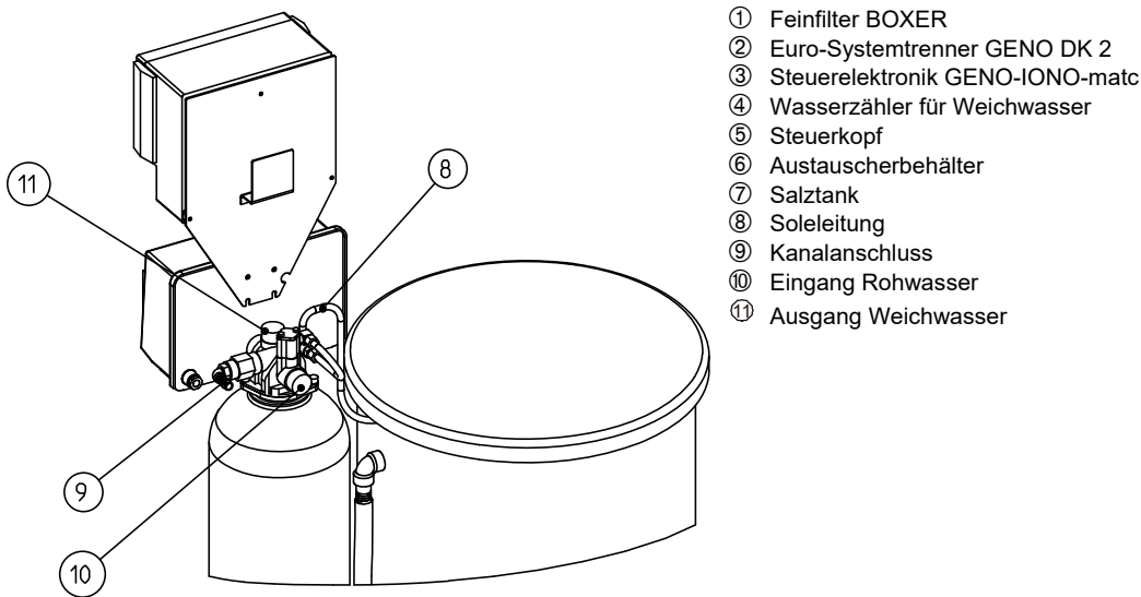
Abb. D-1: (b) Enthärtungsanlage GENO-mat-WF; Hinteransicht
