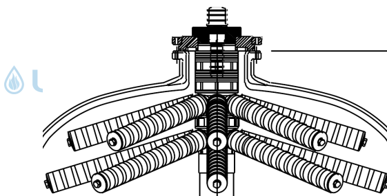
Abb. D-2: Oberes Verteilersystem
