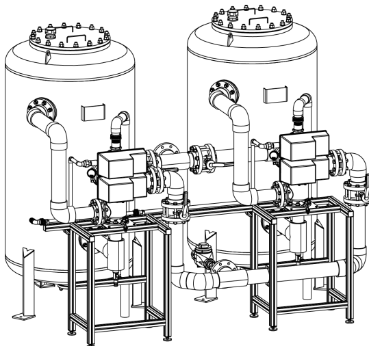
Abb. C-7: Verrohrung mit Absperrklappen
