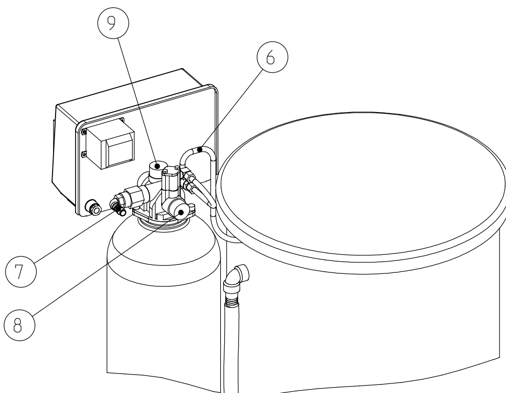
Abb. D-1 (b): Enthärtungsanlage GENO-mat ZF, Hinteransicht
