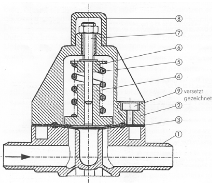
Abb. 1: Schnitt-/Positionszeichnung Überströmventil
