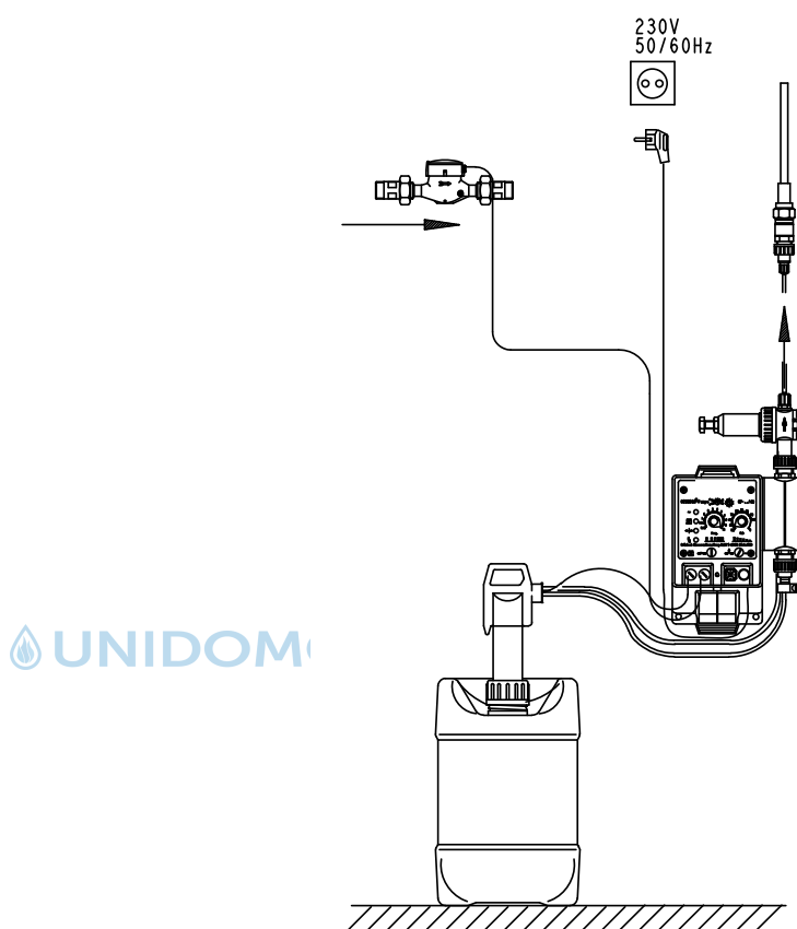
Abb.: Dosieranlage DM-T
