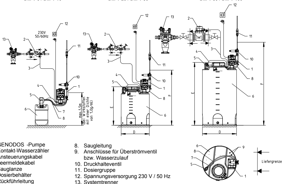
Abb.11.1: Einbauzeichnung DM-T 6 / DM-T 10
