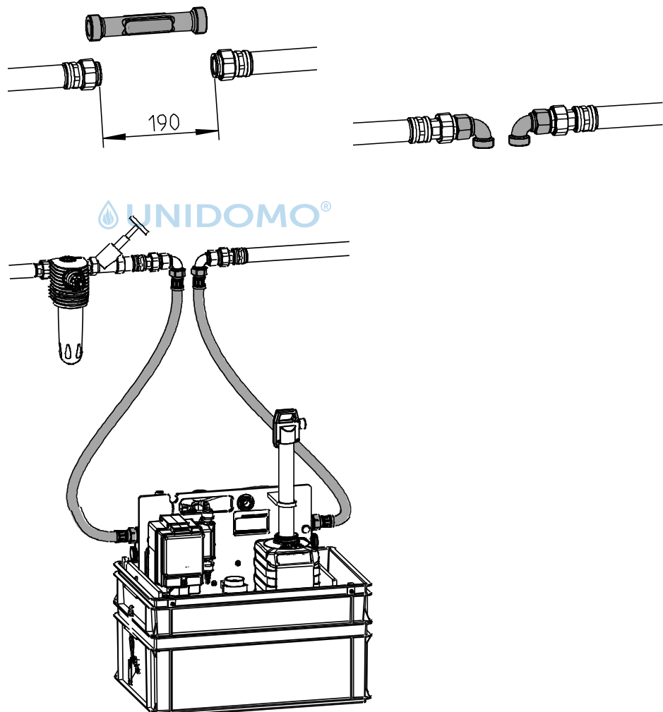
Abb. D-4: Installationsbeispiel Einbindung einer Dosieranlage MOBldos, mit Anschlusswinkel
