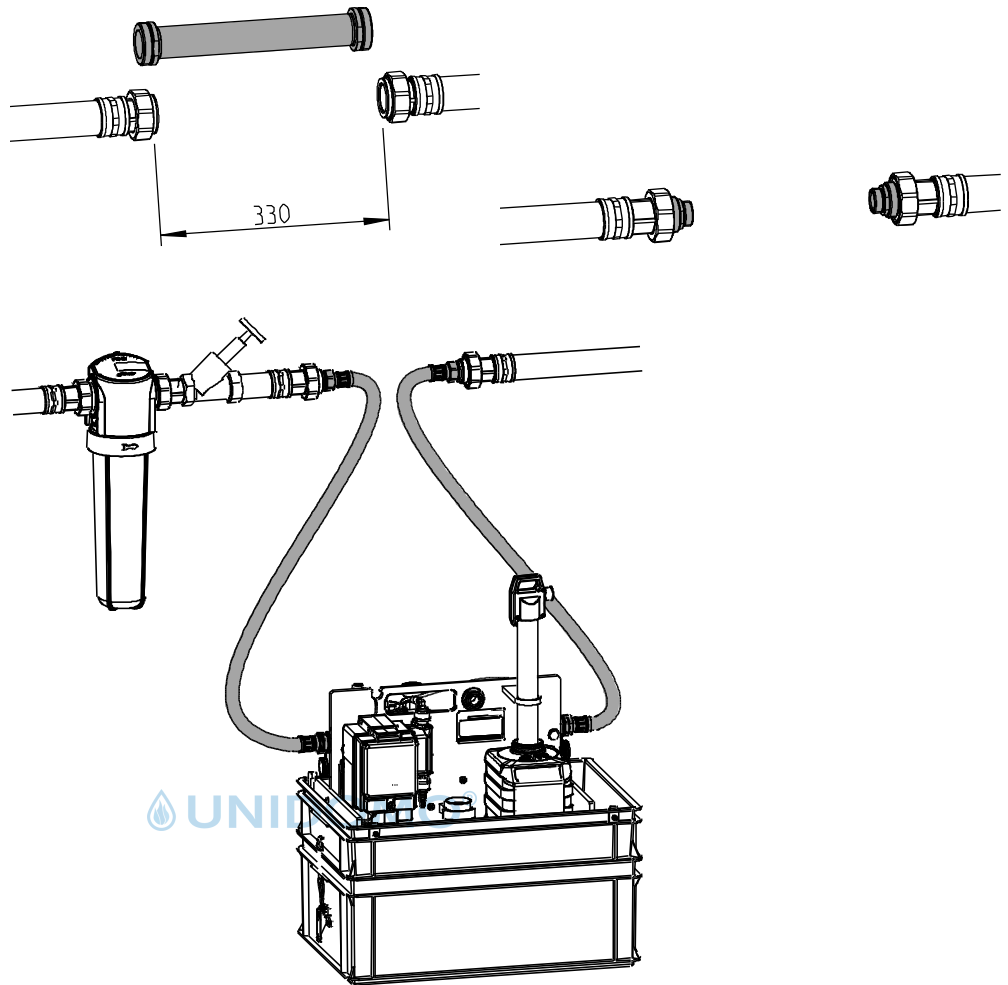
Abb. D-5: Installationsbeispiel Einbindung einer Dosieranlage MOBIdos, ohne Anschlusswinkel
