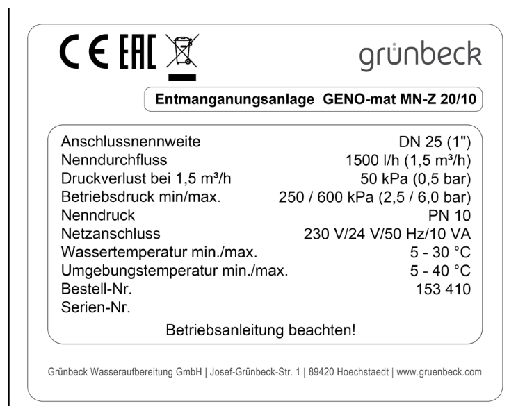
Abb. C-1: Typenschild Enteisenungs-/Entmanganungsanlage GENO-mat MN-Z
