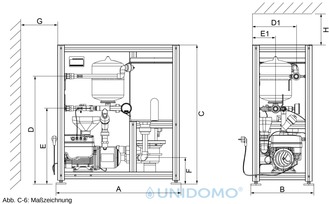
Abb. C-6: Maßzeichnung
