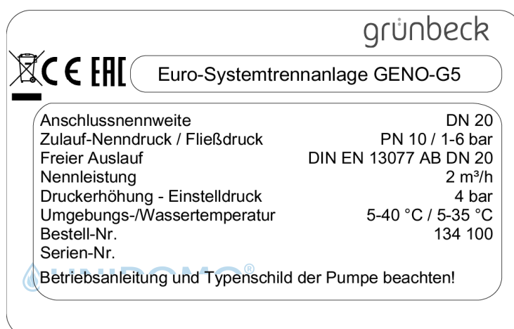
Abb. C-1: Typenschild Euro-Systemtrennanlage GENO-G5
