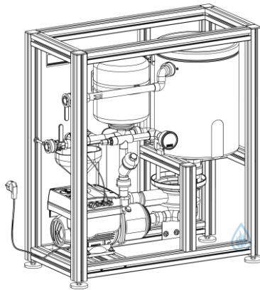
Abb. C-5: Aufbau
