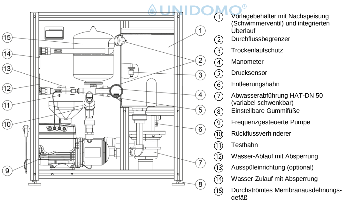
Abb. D-12 Aufbau der Euro-Systemtrennanlage GENO-G5
