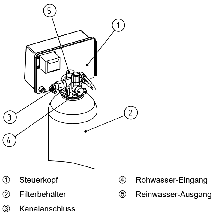
Abb. D-2 (b): Filteranlage GENO-mat, Hinteransicht
