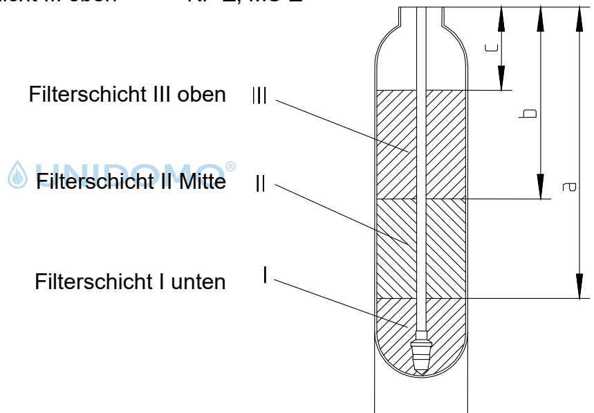
Abb. D-1: Einfüllen der Filterschichten
